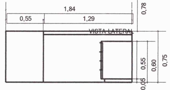
VISTA LATERAL
